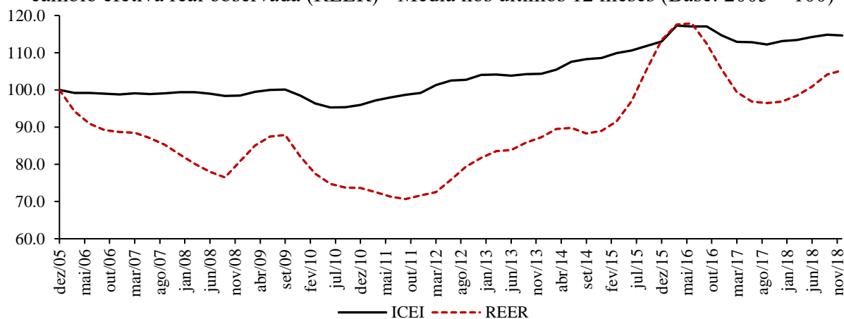
Figura 2. Índice da taxa de câmbio efetiva de equilíbrio industrial (ICEI) e Índice da taxa de câmbio efetiva real observada (REER) - Média nos últimos 12 meses (Base: 2005 = 100)
