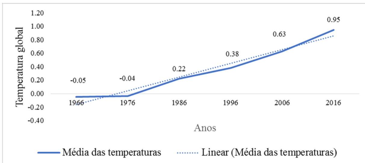
Figura 2 – Crescimento das temperaturas mundiais.
